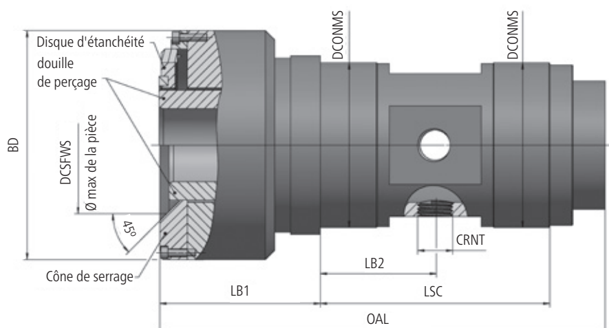
Dimensions de montage
