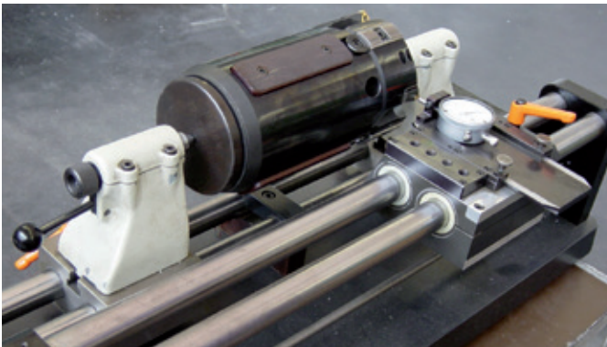
Exemple Type 36 - Montage et réglage cassette
