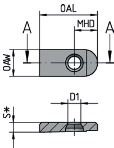
Coupe A-A
